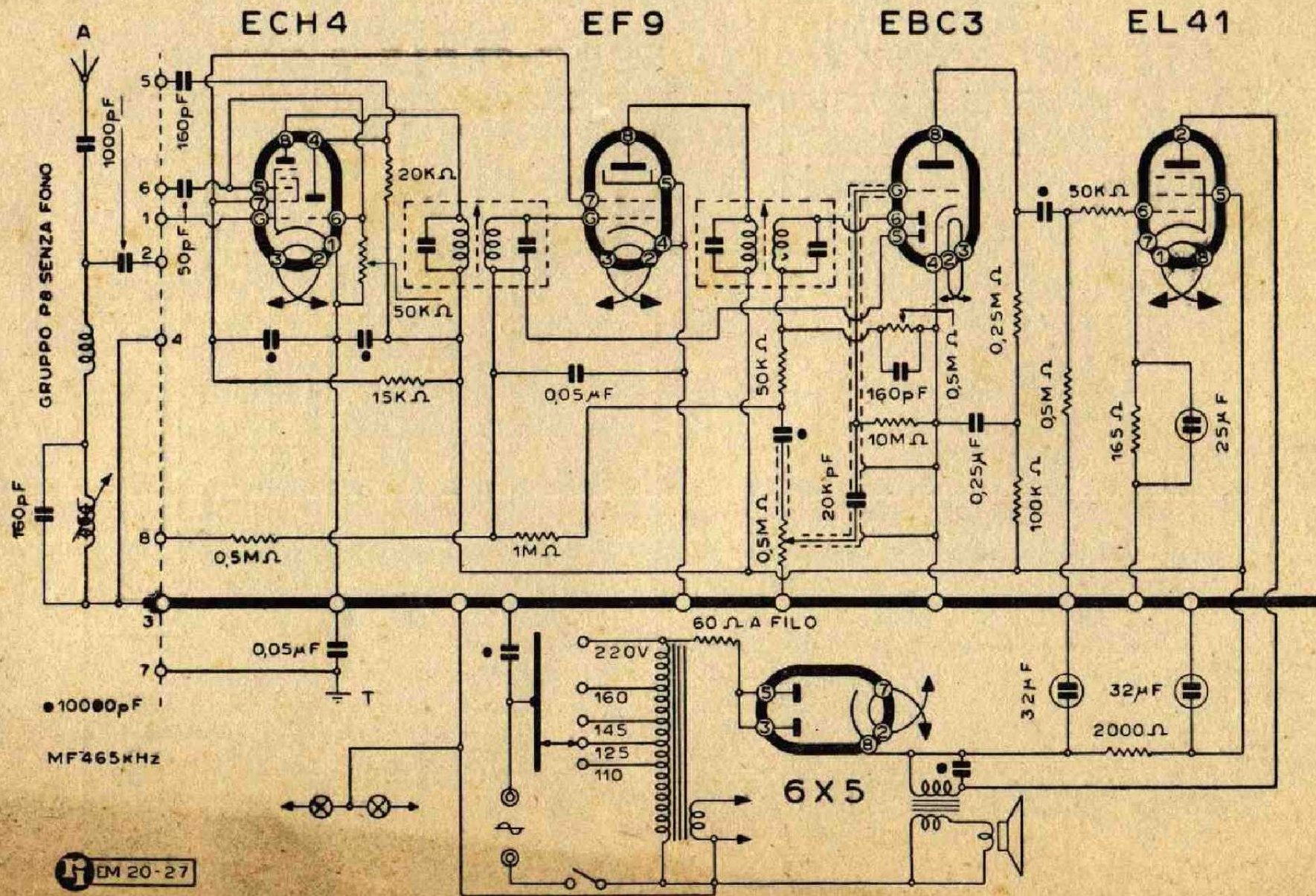
Lo schema elettrico del mod. A2
